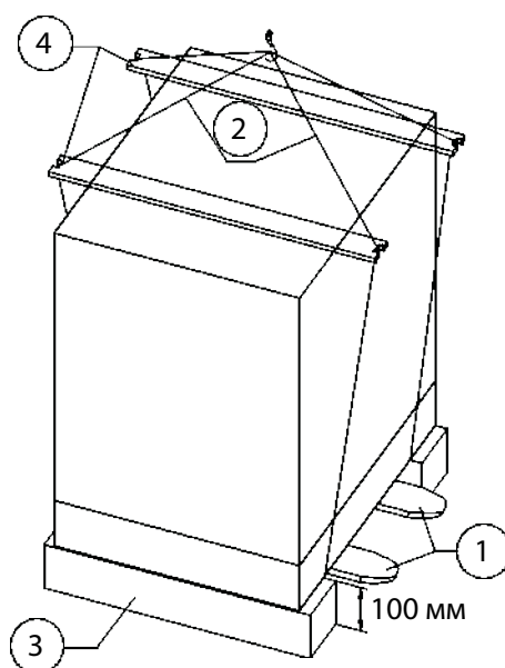
Рисунок 5.1. Схема строповки ККБ моделей 002 – 018
