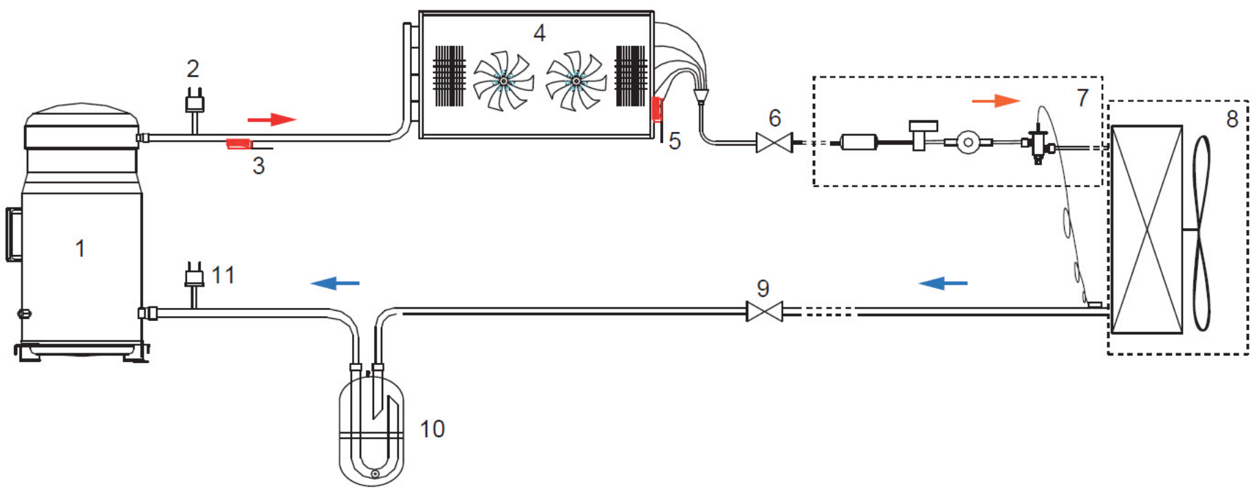
1 — компрессор; 2 — реле высоко давления; 3 — датчик температуры нагнетания; 4 — конденсатор; 5 — датчик температуры трубы конденсатора; 6, 9 — запорный вентиль; 7 — комплект соединительный для ККБ (опция); 8 — секция охлаждения (приобретается отдельно); 10 — отделитель жидкого хладагента; 11 — реле низкого давления
