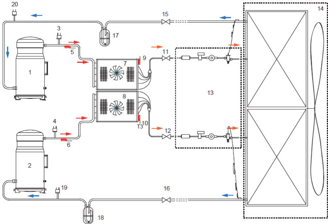
1, 2 — компрессор; 3, 4 — реле высоко давления; 5, 6 — датчик температуры нагнетания; 7, 8 — конденсатор; 9, 10 — датчик температуры трубы конденсатора; 11, 12, 15, 16 — запорный вентиль; 13 — комплект соединительный для ККБ (опция); 14 — секция охлаждения (приобретается отдельно); 17, 18 — отделитель жидкого хладагента; 19, 20 — реле низкого давления
